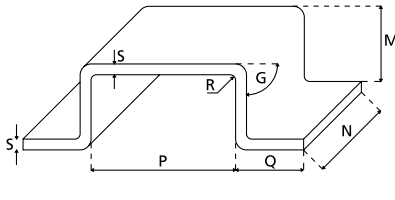
11 = TI PIEGA SCHIACCIATA CON CAM CRUSHED BEND WITH CAM FALTUNG MIT SCHIEBER PLIAGE ÉCRASÉ AVEC CAM
